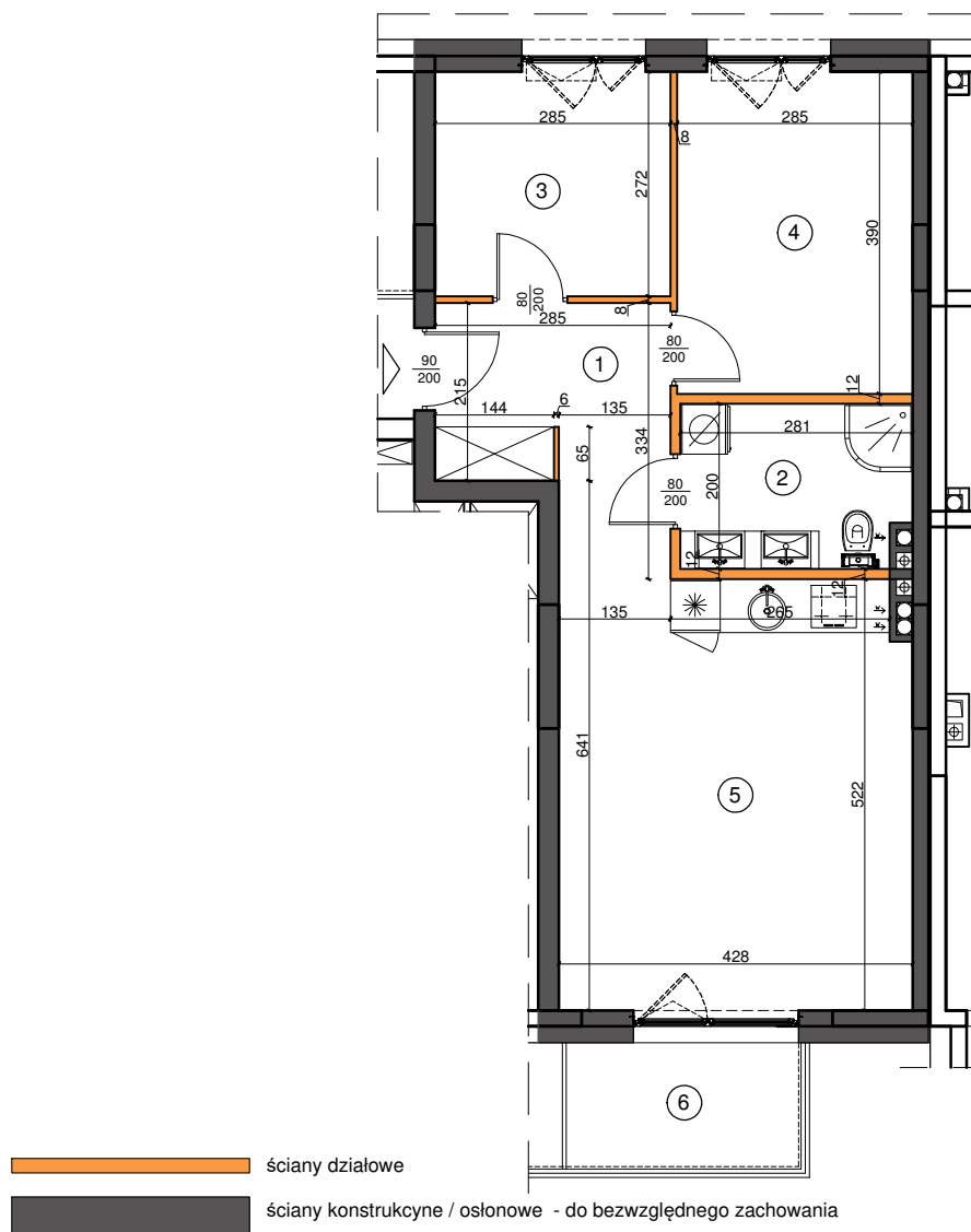
RZUT LOKALU MIESZKALNEGO - SKALA 1:100
